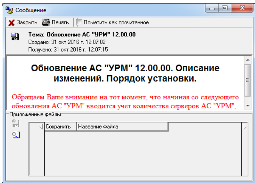
Рис. 10.1. Вид сообщения-напоминания
